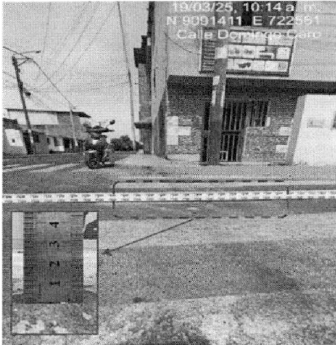
Imagen n.° 12: Depresión de 2,6 cm (regla colocada paralela a la vía) entre unión de la calle Antenor Orrego y calle Alfredo Tello, coordenadas N 9091411 E 722561.
