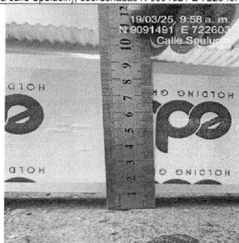
Imagen n.º 25: Depresión de 1,0 cm (regla colocada paralela a la vía) en calle Spelucín, carril derecho (tramo con calle Manuel Arévalo y Antenor Orrego), coordenadas N 9091491 E 722603.
