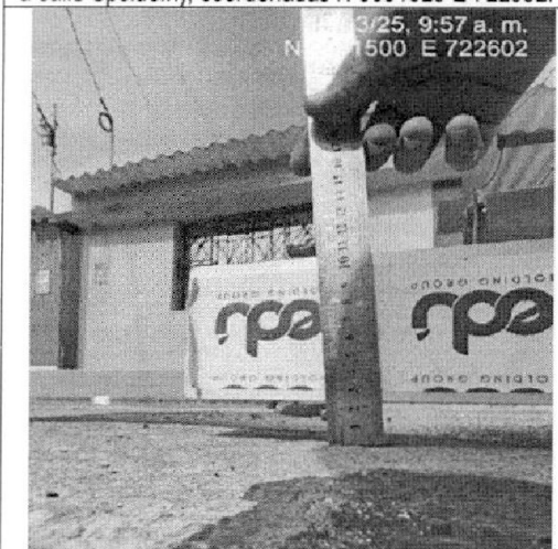
Imagen n.º 24: Depresión de 2,2 cm (regla colocada paralela a la vía) en calle Spelucín, carril derecho (tramo con calle Manuel Arévalo y Antenor Orrego), coordenadas N 9091500 E 722602.
