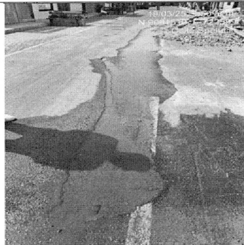
Imagen n.º 27: Deterioro en la capa asfalto en caliente de 2", evidenciándose un bache con acumulación de agua en la calle Spelucín (tramo con calle Manuel Arévalo y Antenor Orrego), coordenadas N 9091510 E 722599.
