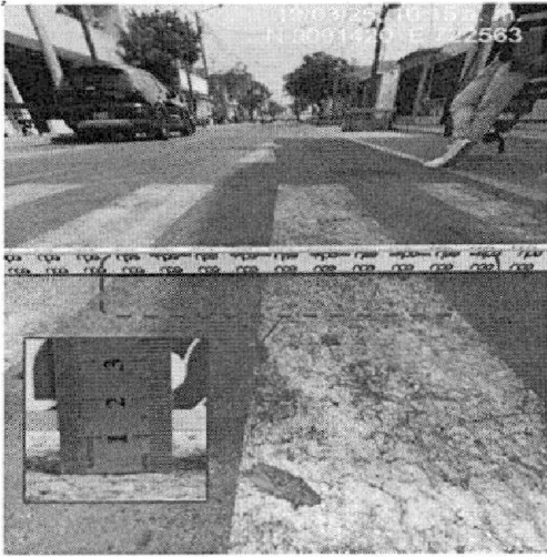
Imagen n.° 13: Depresión de 1,1 cm (regla colocada perpendicular a la vía) en calle Alfredo Tello, carril derecho (entre calle Antenor Orrego y calle Manuel Arévalo), coordenadas N 9091420 E 722563.
