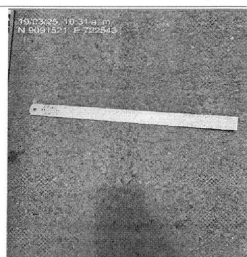
Imagen n.º 23: Presencia de fisuras en la capa asfalto en caliente de 2", carril izquierdo (de calle Alfredo Tello a calle Spelucín), coordenadas N 9091521 E 722543.
