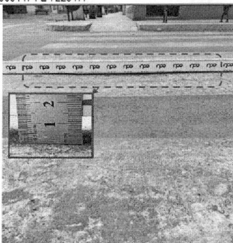
Imagen n.º 20: Depresión de 1,3 cm (regla colocada paralela a la vía) en calle Manuel Arévalo coordenadas N 9091535 E 722580.
