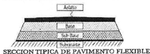
SECCION TIPICA DE PAVIMENTO FLEXIBLE
