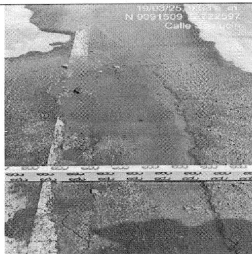
Imagen n.º 28: Deterioro en la capa asfalto en caliente de 2", evidenciándose un bache con presencia de agua en la calle Spelucín (tramo con calle Manuel Arévalo y Antenor Orrego), coordenadas N 9091510 E 722597.
