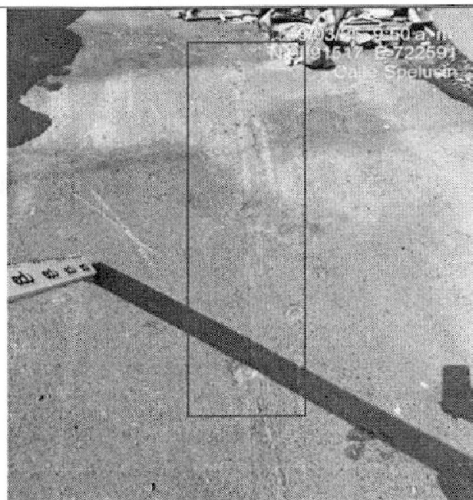
Imagen n.º 26: Deterioro en la capa asfalto en caliente de 2", calle Spelucín (tramo con calle Manuel Arévalo y Antenor Orrego), coordenadas N 9091517 E 722591.
