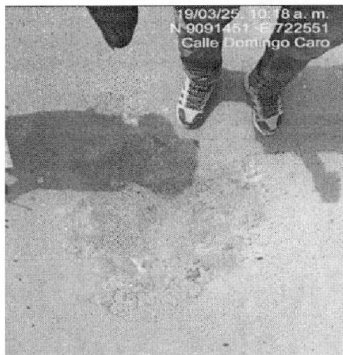
Imagen n.º 16: Peladura de la capa de asfalto en caliente de 2", en calle Alfredo Tello, en coordenadas N 9091451 E 722551.
